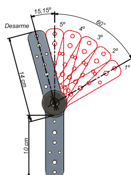
C24605 CATRACA BLINDADA 60° com 5 POSIÇÕES
