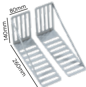
FRA006 - FRAMER 400x80x1,8 C/ TRAVA - PINTADO
