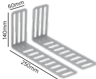
FRA051 - FRAMER 390x60x2,65 S/ TRAVA (140x250) - GALVANIZADO
