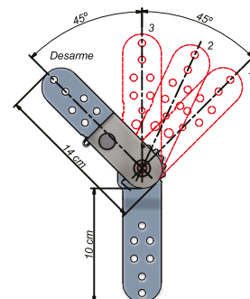
C24413 CATRACA SLIM 45° com 3 POSIÇÕES
