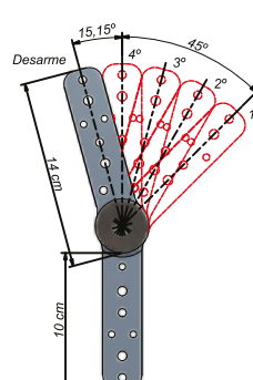
C24454 CATRACA BLINDADA 45° com 4 POSIÇÕES
