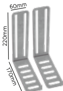
FRA072 - FRAMER 390x60x2,65 S/ TRAVA (220x170) - GALVANIZADO
