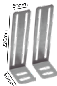
FRA027 - FRAMER 300x60x2,65 S/ TRAVA (220x80) - GALVANIZADO
