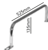
ALC009 - SUPORTE TUBO 5/8 FIX. LATERAL BEGE ALC030 - SUPORTE TUBO 5/8 FIX. LATERAL BLACK ALC008 - SUPORTE TUBO 5/8 FIX. CROMADA
