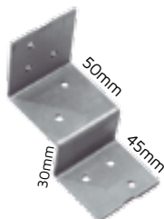
SUL040 - SUPORTE P/ POLTRONAS
