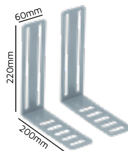
FRA070 - FRAMER 420x60x2,65 S/ TRAVA (220x200) - GALVANIZADO
