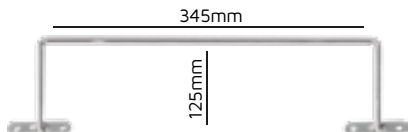
ALC003 - SUPORTE FERRO 1/4 FIX. LATERAL BEGE ALC022 - SUPORTE FERRO 1/4 FIX. LATERAL BLACK ALC018 - SUPORTE FERRO 1/4 FIX. CROMADA
