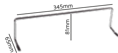
ALC016 - SUPORTE FERRO 1/4 FIX. POR CIMA BEGE ALC023 - SUPORTE FERRO 1/4 FIX. POR CIMA BLACK ALC017 - SUPORTE FERRO 1/4 FIX. POR CIMA CROMADA
