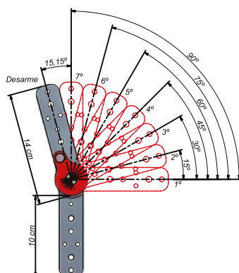
C24902 RETORNO AUTOMÁTICO 90° com 7 POSIÇÕES
