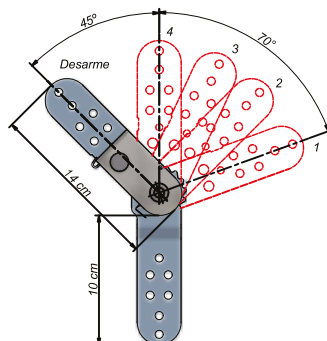
C24713 CATRACA SLIM 70° com 4 POSIÇÕES
