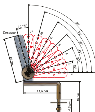
C24904 - CATRACA BLINDADA BRAÇO PRETO FOSCO 90° com 7 POSIÇÕES
