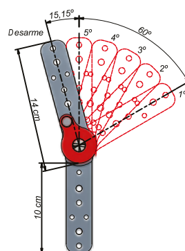
C24602 RETORNO AUTOMÁTICO 60° com 5 POSIÇÕES
