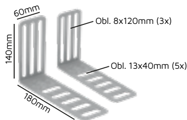
FRA075 - FRAMER 320x60x2,65 S/ TRAVA (140x180) - GALVANIZADO
