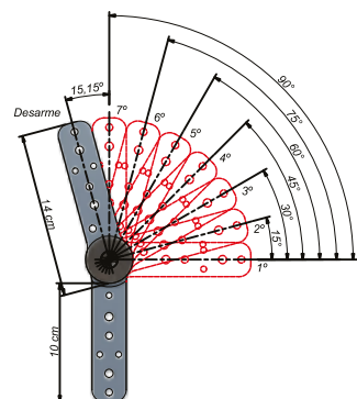
C24907 CATRACA BLINDADA 90° com 7 POSIÇÕES
