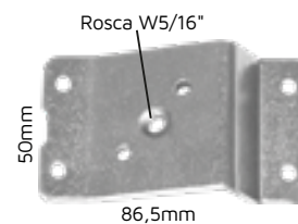
SUL011 - SUPORTE P/ PÉ DE POLTRONAS 2,65mm C/ ROSCA
