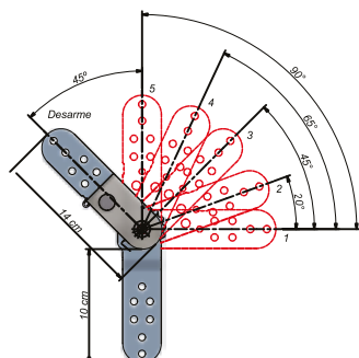
C24913 CATRACA SLIM 90° com 5 POSIÇÕES
